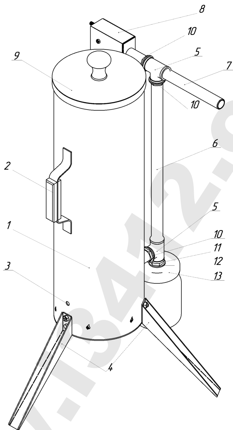
Рисунок 1 — Дымогенератор ВОРОН NEW 10 л
