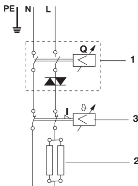
Рис. 5. NPX Aquatronic DIGITAL 2.0
