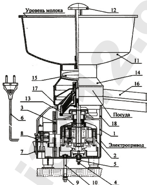
Рисунок 1 – Устройство сепаратора
