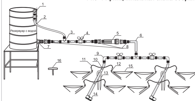
Рис. 1 Принципиальная схема сборки
